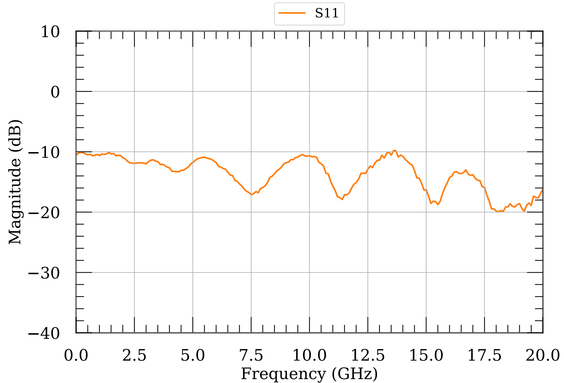
LNA S-params module065v2
